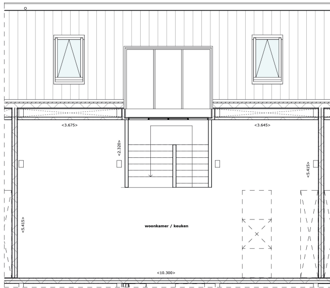
Plattegrond verdieping 04 1:50
