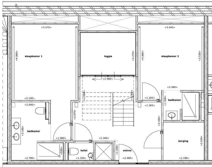
Plattegrond verdieping 03 1:50
